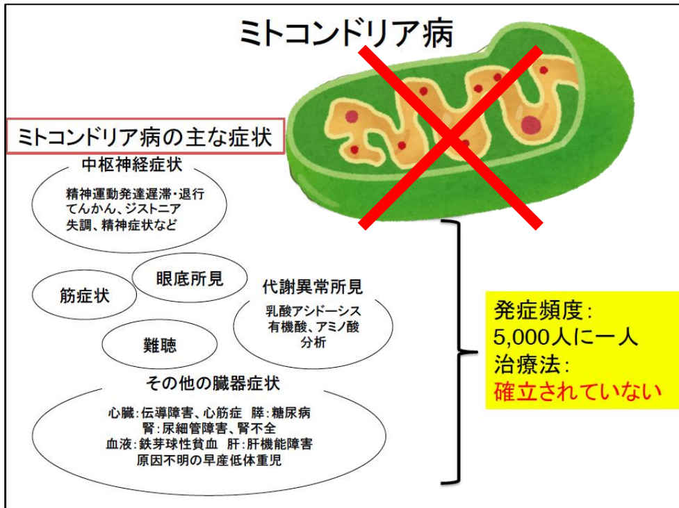
図1. ミトコンドリア病
