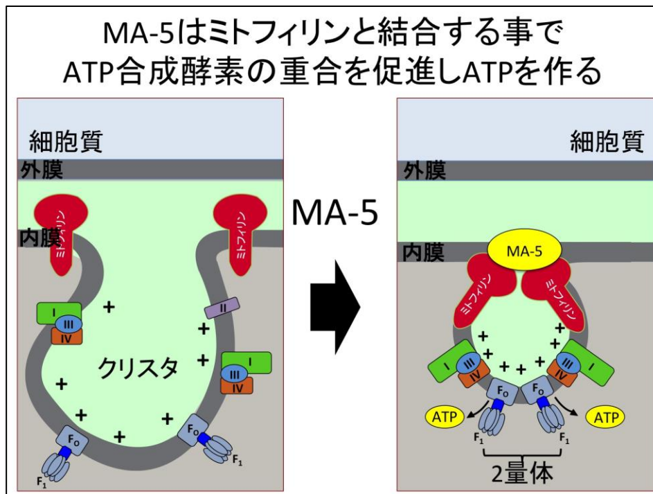
図2. ATP合成の新たなメカニズム
