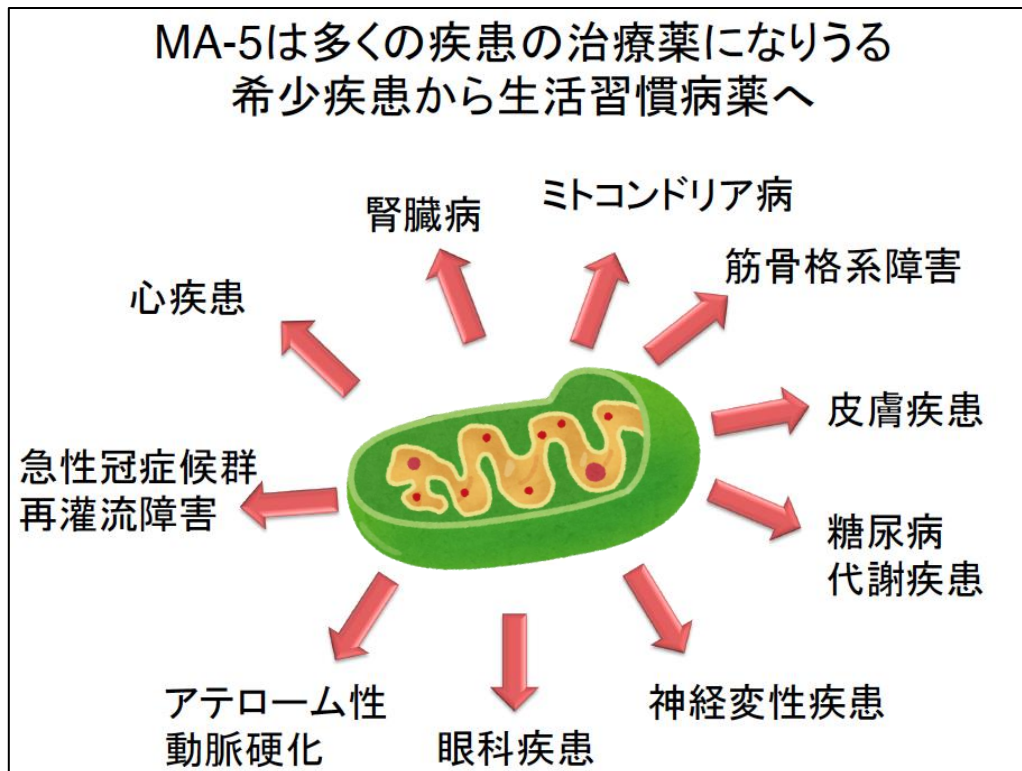
図5. MA-5は多くの疾患の治療薬となる可能性がある
