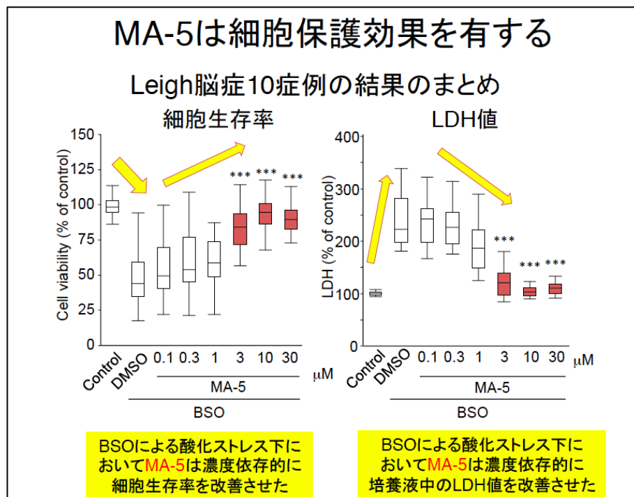
図4. MA-5による細胞保護効果
