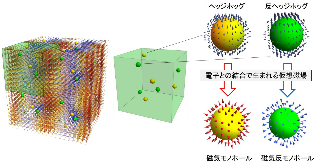
図1 MnGe におけるトポジカル磁気構造体 (ヘッジホッグ・反ヘッジホッグ) とそれらが電子に与える仮想磁場の分布 (磁気モノポール・反モノポール)
