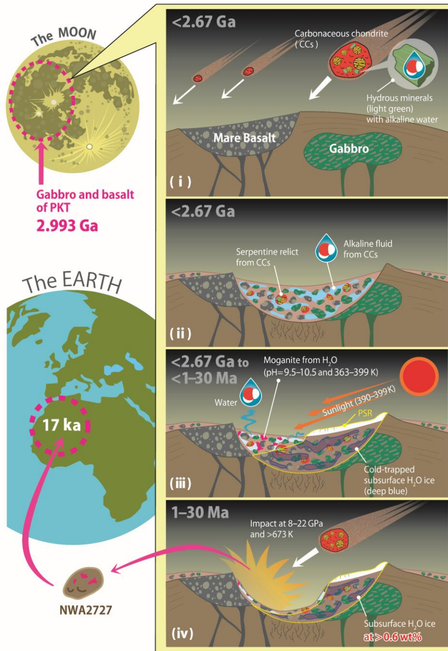
図 4: 月への水の供給とモガナイトの沈殿の概念図。① 約 30 億年前に月のプロセルム盆地で月隕石の母体となる深成岩体 (Gabbro と Mare Basalt) がマグマから固化、② 27 億年前以降にプロセルム盆地にアルカリ性の水を豊富に含む炭素質コンドライト (Carbonaceous chondrite) が衝突、③ 衝突で形成したクレーターの一部が、放出された月の地殻の一部や炭素質コンドライトの破片で埋まり、その後の角礫化作用によってクレーターの表面から底部にかけて水が捕縛、④ 太陽光が当たる表面では水が蒸発してモガナイトを沈殿、低温の地下や影では水が氷となり (1 億 3000 万年前?)、その埋蔵量は 0.6 wt%、⑤ 100-3000 万年前までに巨大天体の衝突でクレーターの一部の岩石が宇宙に放出、⑥ 宇宙を漂って 1 万 7000 年前に地球の北西アフリカの砂漠に月隕石として落下 (illustrated by M. Sasaoka (SASAMI-GEO-SCIENCE))
