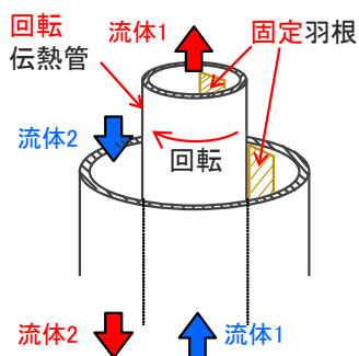
図1 開発した回転式熱交換器(概略)
