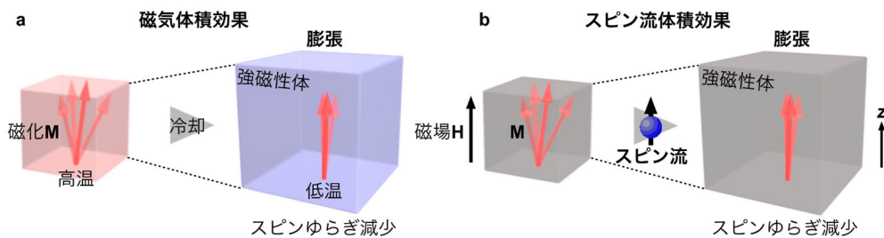
図1：磁気体積効果とスピン流体積効果の模式図
