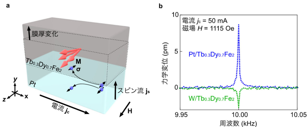
図2：スピン流体積効果測定の様式図およびスピン流注入に対する \text{Tb}_{0.3}\text{Dy}_{0.7}\text{Fe}_2 の力学応答測定結果
