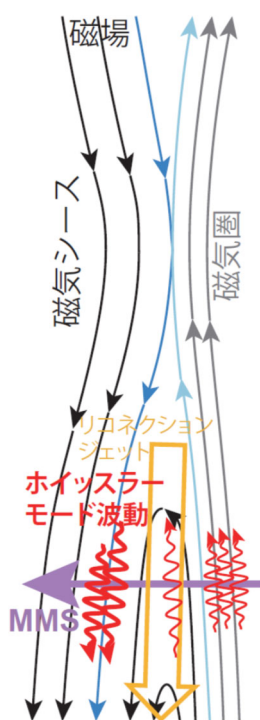
図 3、磁気リコネクションと観測領域(反平行な磁場のつなぎ変わりによって生じる磁気リコネクションの南側で、リコネクションによるプラズマの高速な流れ(リコネクションジェット)と磁気シース領域の境界付近で観測された波動と電子の相互作用について解析を行った。) (Kitamura et al. Nature Comm., 2022 の論文の図を一部変更し日本語説明を加筆)
