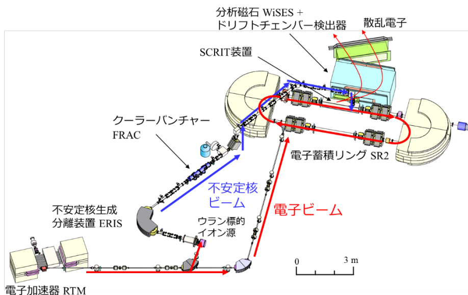
図 2 SCRIT 電子散乱施設
