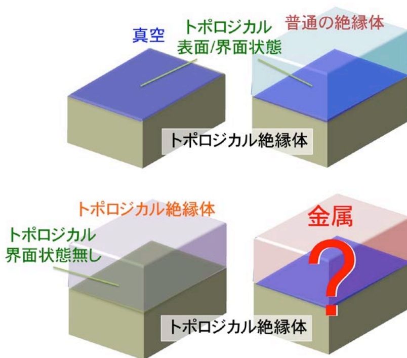
図2: トポジカル絶縁体と絶縁体・金属の接合. 絶縁体との接合に比べて, 金属との接合はこれまで研究例が殆ど無い.
