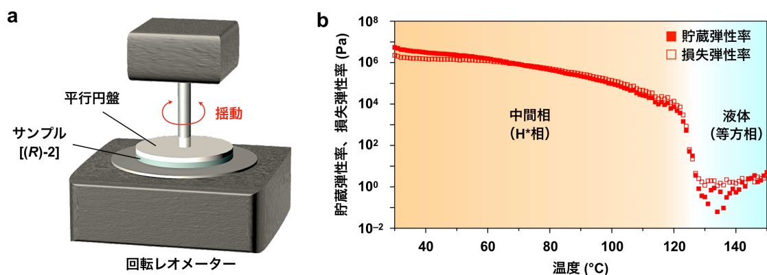
図 3. (a) 回転レオメーターを用いた (b) 温度可変動的粘弾性測定の結果
