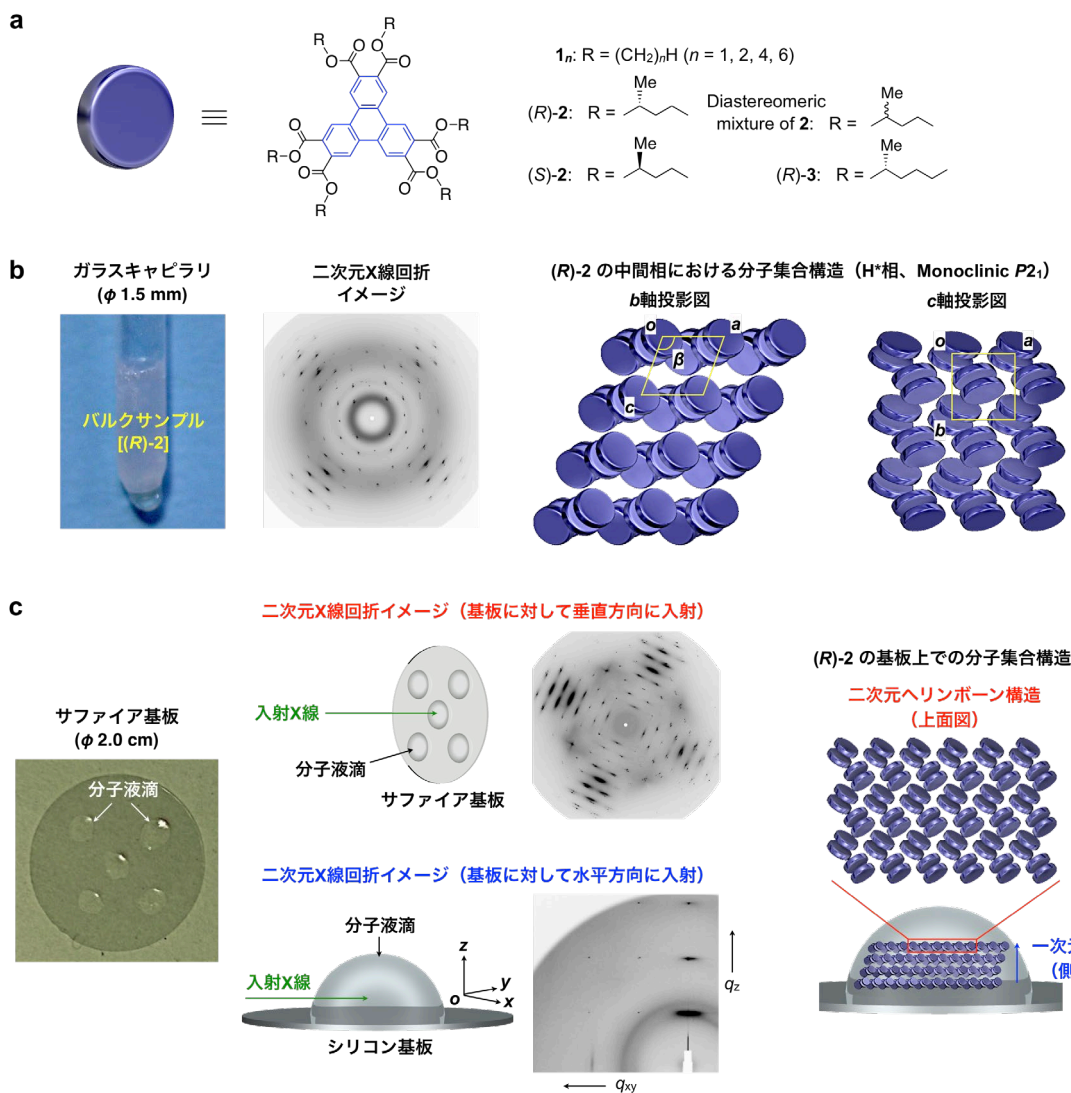
図 1. (a) キラルトリフェニレンの分子構造、(b) 液滴中の分子集合構造、および (c) 基板上での液滴内部の分子集合構造
