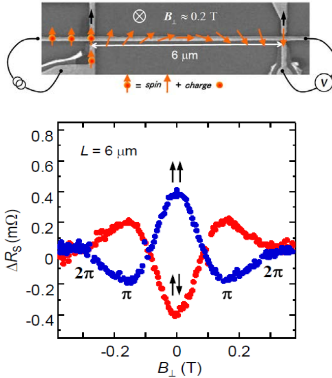
図 4 ハンル効果を用いたスピン歳差運動の実験概念図と実験結果
