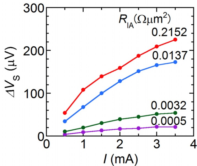
図3 磁気蓄積素子の出力電圧の印加電流依存性
