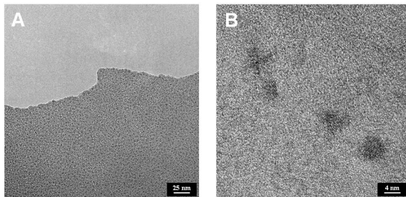
図 2. 試料ガラスを熱処理することで得られたナノメトリック相分離 (A) と NaNbO 3 ナノ結晶 (B).
