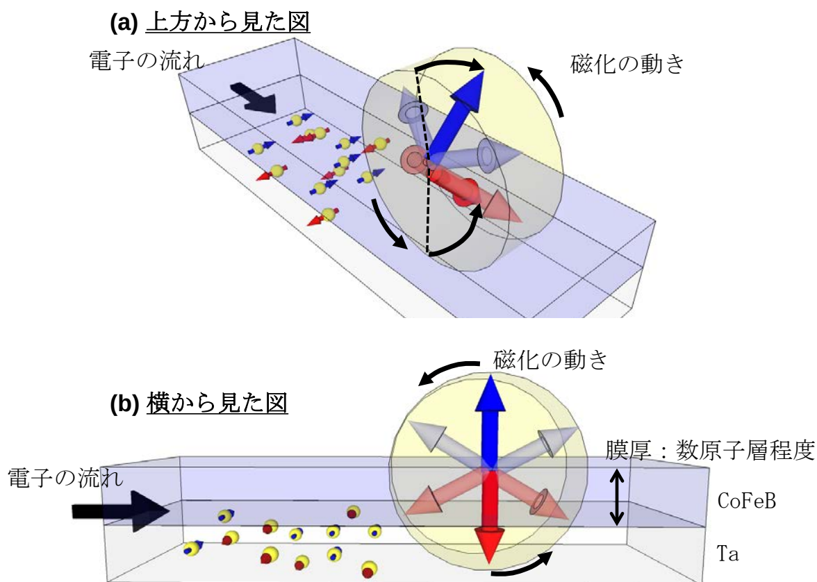
図3. Ta/CoFeB/MgO 磁性ナノヘテロ接合に電流を流した際の磁化の動きを模式的に表したもの。スピンホール効果などによってスピンの流れが生成され、その一部が磁性層に進入すると、磁性層の磁化にトルクが作用する。今回、トルクが作用する方向や大きさを調べ、電流と平行な成分と直交する成分が存在することを発見した。電流を流していない時、磁化は膜面垂直方向を向いている。電流を流すと、磁化が面内方向に傾く ((a)図参照) のと同時に回転 ((b)図参照) を始める。イメージとして、水車の軸を磁化、水車を駆動する水を電子の流れとするとわかりやすい (実際に磁化が傾斜、回転する機構は、様々な効果が絡んだより複合的なものである。)
