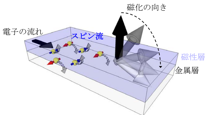
図 2. スピンホール効果を利用した磁化反転の模式図。ここでは例として、非磁性層／磁性層の 2 層膜において、電流を膜面水平方向に流すだけで磁化反転が誘起されることを模式的に表した。上図では、すべての電子は電界印加によって右方向に移動するが、スピンホール効果によって、青スピンは上に、赤スピンは下に動く。磁性層に進入した青スピン（スピンの流）が十分な大きさになると、磁性層の磁化が反転する。反転した磁化を元に戻すには、電流の向きを変えればよい。
