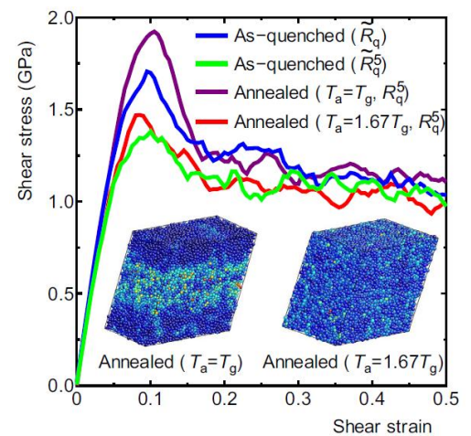
図 1 構造若返りによる金属ガラスモデルの変形特性の変化: 構造若返りが起きた右のモデルでは変形がより均一に生じるようになる。
