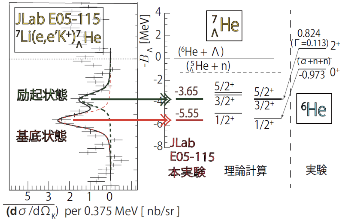
図 3: 測定された {}^7_{\Lambda}\text{He} ハイパー核のラムダ粒子束縛エネルギースペクトラムと観測された基底状態（赤線）、励起状態（緑線）のエネルギー準位を示します。本研究により測定されたラムダ粒子束縛エネルギーの隣に 2 種類の理論予想と芯核である {}^6\text{He} のエネルギー準位を示しました。 {}^6\text{He} にラムダ粒子を付け加え {}^7_{\Lambda}\text{He} ハイパー核とすることでラムダ粒子の「糊的役割」が働き、より深く束縛していることが分かります。
