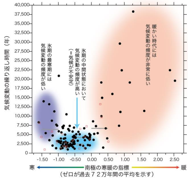
図 3：南極アイスコアの解析から得られた、過去 72 万年間における気候変動の繰り返し時間（頻度）と南極の気温との関係（黒丸）。グリーンランドのアイスコアによる最終氷期の結果も示す（赤四角）。間氷期のような暖かい時代や、氷期の最寒期のような寒い時代には頻度が低い、氷期の間状態の寒さの時代に気候変動が頻繁に起こっており、気候が不安定であったことが示された。
