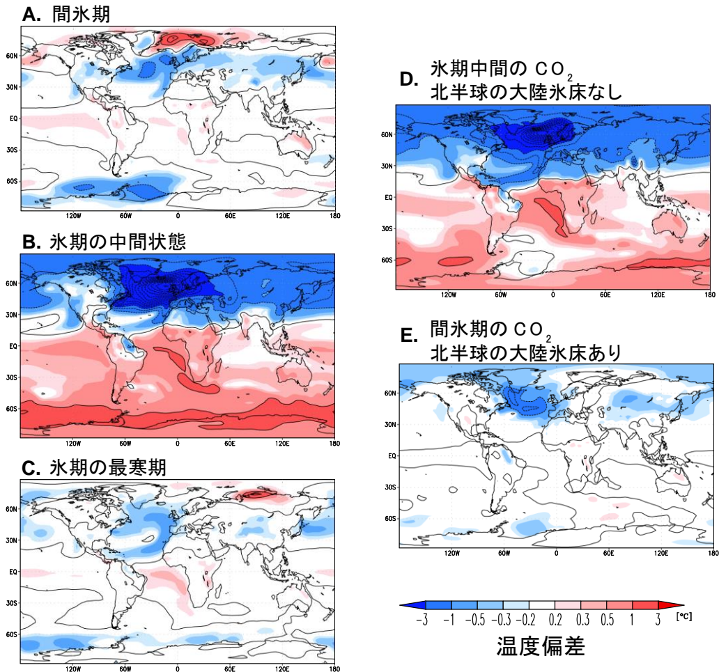
図 4：大気海洋結合大循環モデル (MIROC) による気候シミュレーションの結果。(A-C) まず3つの異なる気候状態を再現した(間氷期、氷期中間状態、氷期最寒期のそれぞれに相当する大気中二酸化炭素濃度と氷床形状を与えた)。その後、北大西洋北部に淡水を500年間加え続けた後の初期状態からの温度偏差を示す。氷期中間状態の時に反応が大きく、北半球が寒冷化し、南半球は逆に温暖化することが分かる。(D, E) 現実には存在しなかった条件下での感度実験の結果。間氷期の条件から、大気中二酸化炭素濃度または北半球氷床のみを氷期中間状態と同じにした。その結果、気候の不安定性が増大する要因として大気中二酸化炭素の役割が大きいことが分かった。
