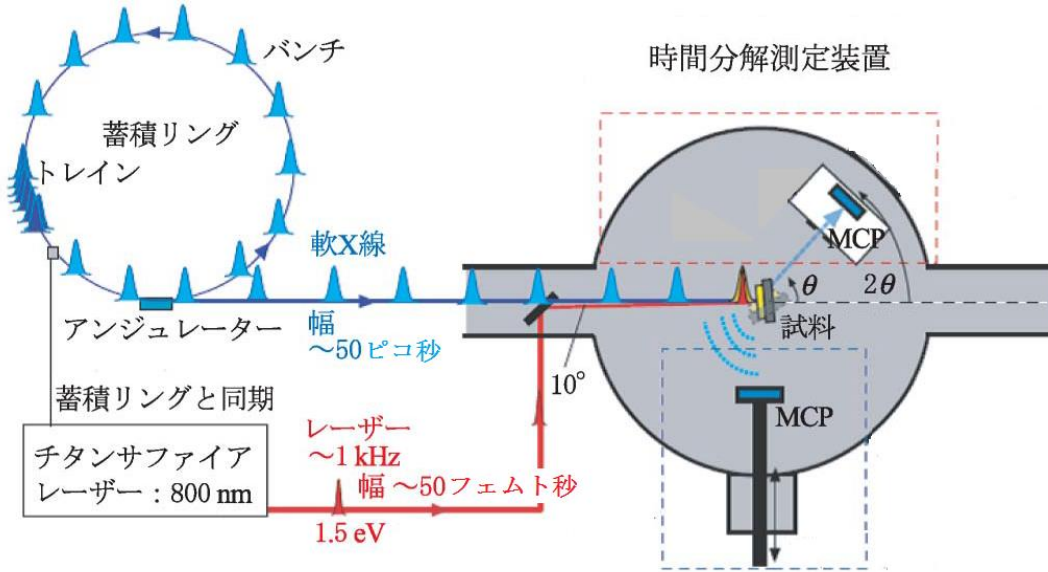
図1：時間分解 XMCD 測定の設定アップ。
