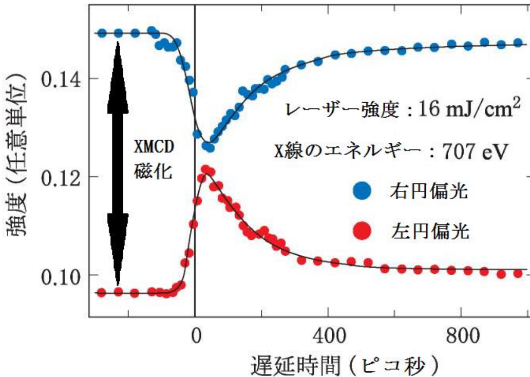
図2：時間分解 XMCD 測定で観測された磁化の時間変化の様子。
