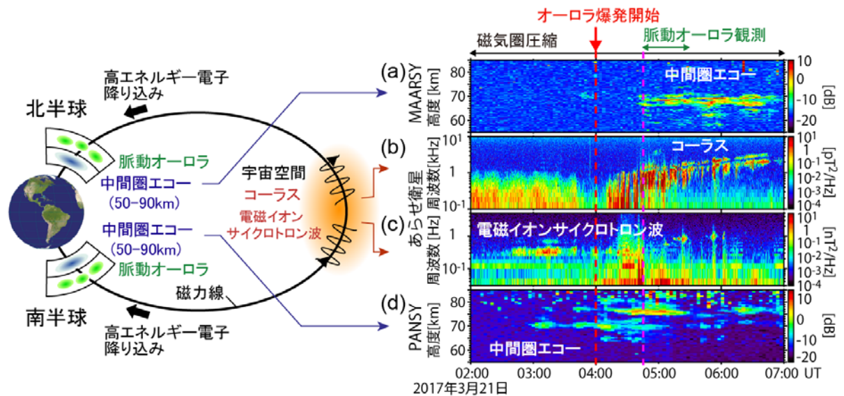
図 2: 2017 年 3 月 21 日 02~07 時に、あらせ衛星で観測された地球周辺の宇宙空間の電磁波と、南北極域の大型大気レーダーPANSY、MAARSY で観測された中間圏エコー。(a) ノルウェーの MAARSY レーダーで観測された高度 55~85km からの反射エコー強度。(b) あらせが観測した高周波帯(0.1~10kHz)、(c) 低周波帯(0.03~5Hz)の電磁波の強度。(d) 南極昭和基地の PANSY レーダーで観測された高度 55~85km からの反射エコー強度。(b)、(c)で、あらせが電磁イオンサイクロトロン波(2:30~4:45)、コーラス(4:45~7:00)を観測した時間帯に、(a)、(d)で、南北両半球のレーダーが中間圏エコーを観測した。
