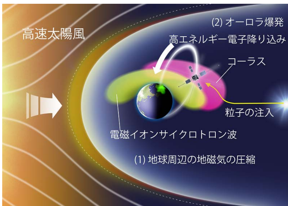
図 4: 高エネルギー電子が大気へ降り込む過程のイメージ。(1)太陽から吹く高速太陽風が地球周辺の地磁気を圧縮し、電磁イオンサイクロトロン波を成長させ、その後、(2)オーロラ爆発が発生し、宇宙空間夜側から熱い電子が朝側に運ばれ、コーラスを発生させた。これらの電磁波が宇宙空間の高エネルギー電子を磁力線に沿って極域大気に落とし、上層でオーロラを、下層で中間圏の大気電離を引き起こしたと考えられる。
