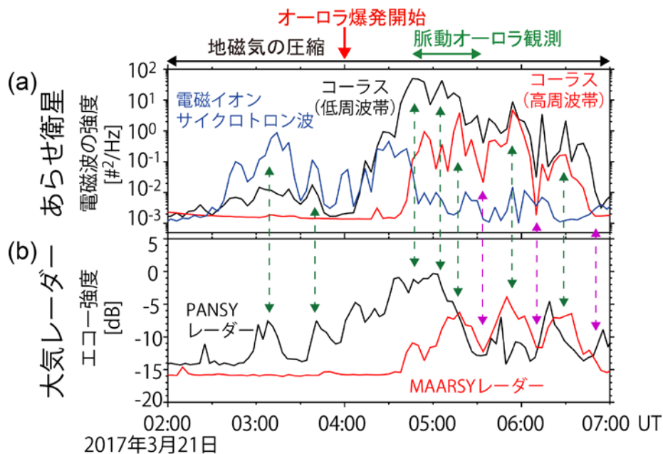
図 3: (a) あらせ衛星が観測した電磁波の強度の時間変化。電磁イオンサイクロトロン波は卓越周波数帯(0.2~0.5Hz)における平均値を、コーラスは高周波帯と低周波帯に分け、それぞれの周波
