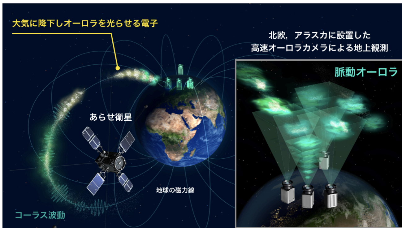
図 1: (左) コーラス波動によってジオスペースの電子が叩き落とされ、磁力線に沿って地球大気へ降下し、オーロラを光らせる様子。(右) 本研究によって北欧とアラスカに設置された高速オーロラカメラによる観測の模式図。
