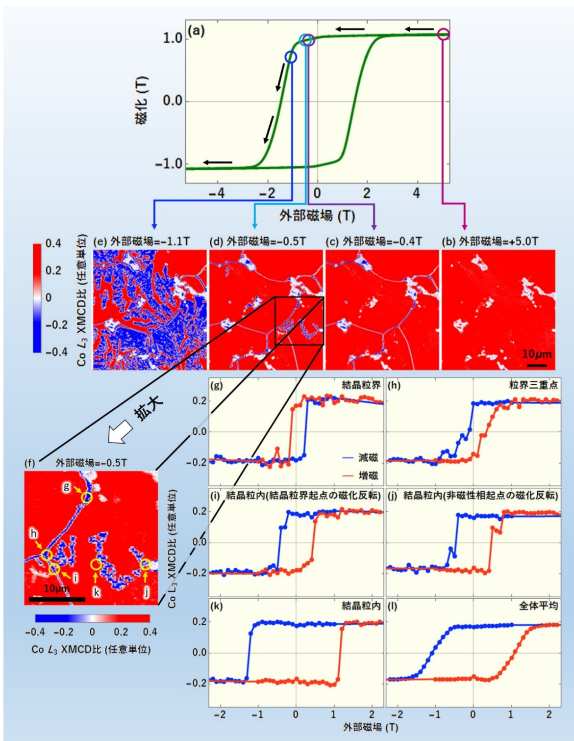
図1 異方性 (\text{Sm, Ce})_2(\text{Co, Fe, Cu, Zr})_{17} 磁石のバルク磁化曲線(a)。Co L_3 XMCD 比を用いた磁区像の外部磁場依存性、外部磁場 +5.0\text{ T} (b)、 -0.4\text{ T} (c)、 -0.5\text{ T} (d)、 -1.1\text{ T} (e)。結晶粒内に磁化反転が進展した領域の拡大図 (f)。磁化曲線の場所依存性、結晶粒界(g)、粒界三重点(h)、結晶粒界から結晶粒内に向かって磁化反転が進展した位置(i)、非磁性相から結晶粒内に向かって磁化反転が進展した位置(j)、結晶粒内(k)、局所磁化曲線の全体平均(l)。
