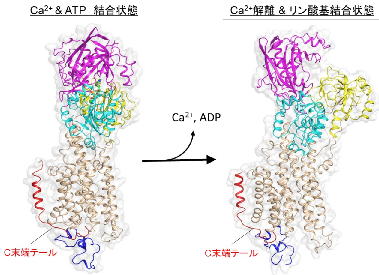
図 2 SERCA2b の二つの中間状態のクライオ電子顕微鏡構造
