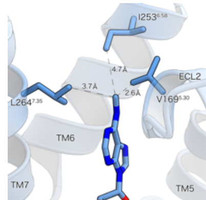
図5 予測されたm 6 AとアデノシンA3受容体の結合様式
