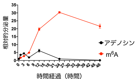
図3 m 6 Aとアデノシンは細胞障害時に異なる分泌パターンを示す
