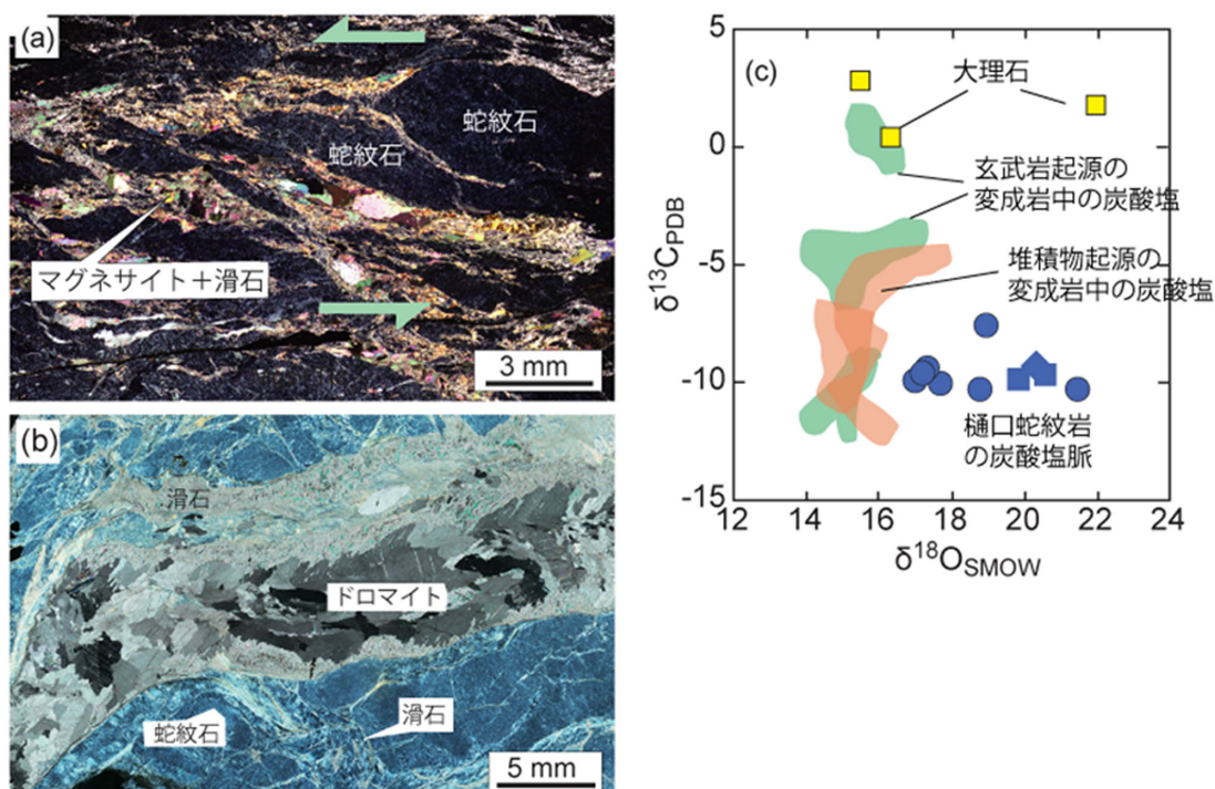
図 2 樋口蛇紋岩体の炭酸塩脈の特徴。(a) 蛇紋石 (アンチゴライト) のブロックを切るマグネサイト+滑石脈。蛇紋石ブロックの非対称の組織から剪断変形を受けていることがわかる。(b) ドロマイト+滑石脈。蛇紋石と二酸化炭素が反応する炭酸塩化反応では、シリカが放出されるために、シリカに富む層状ケイ酸塩鉱物である滑石ができる。滑石は変形しやすいやわらかい鉱物であり、プレート境界の性質を大きく変化させる。(c) 樋口蛇紋岩体の炭酸塩鉱物の炭素と酸素の安定同位体組成。三波川帯の中に出てくる大理石 (海洋底で形成した炭酸塩が沈み込んだもの) とは大きく異なっている。蛇紋岩中の炭酸塩脈の炭素同位体は、堆積物起源の变成岩に含まれる炭酸塩とよく似ているが、酸素同位体はより高くなっており、堆積物中の炭素を起源とする二酸化炭素と蛇紋岩から脱水した水が混合したことを示唆している。
