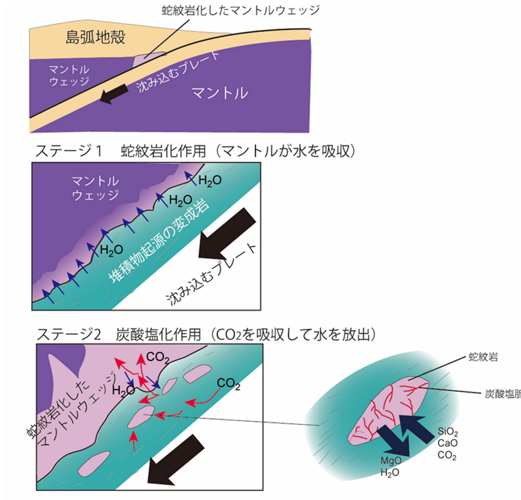
図3 沈み込み帯のマントルでの炭酸塩化作用の模式図。沈み込むプレートとマントルウェッジの先端は蛇紋岩化していると考えられている。
