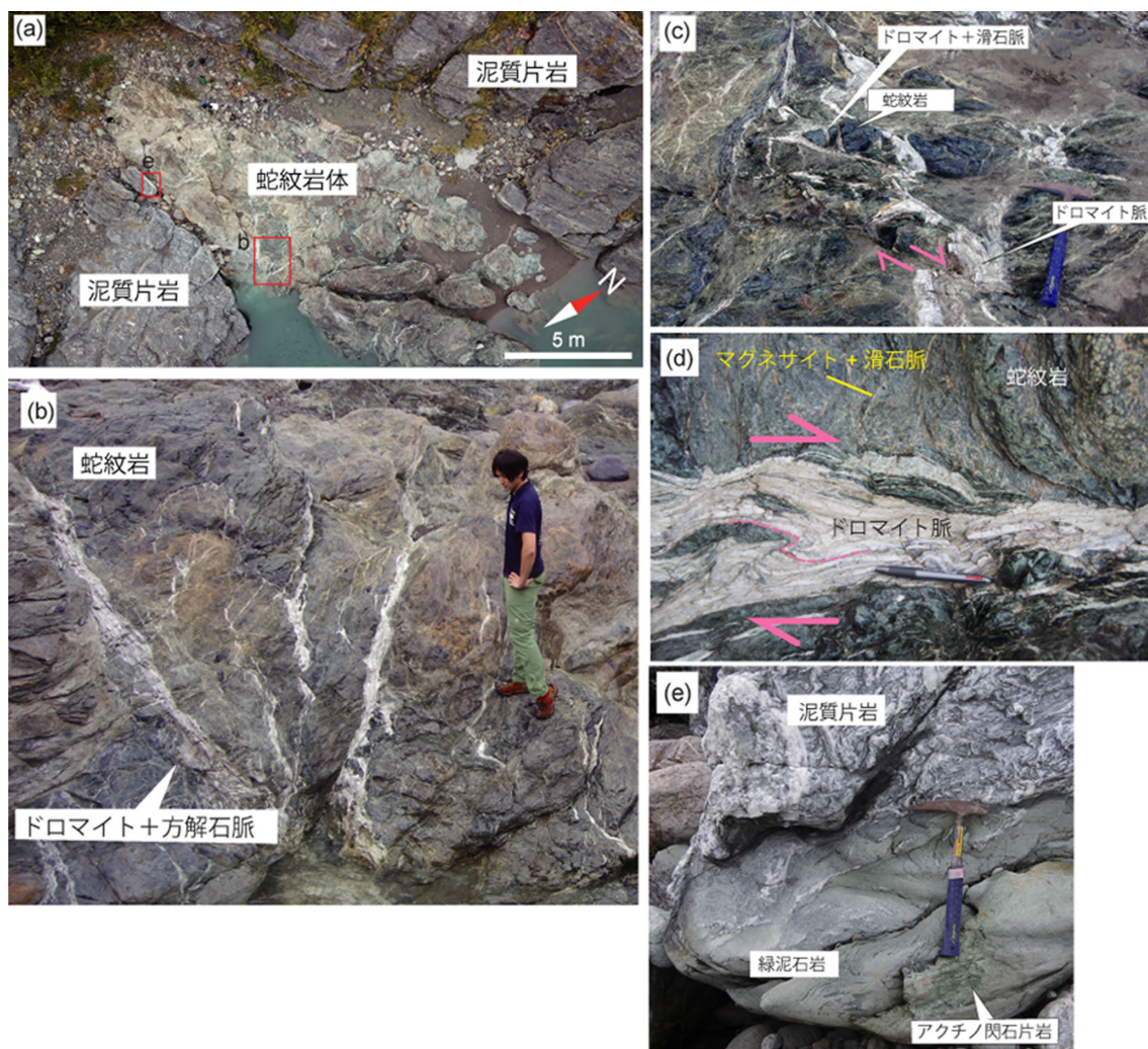
図 1 露頭における樋口蛇紋岩体と炭酸塩脈(き裂を炭酸塩鉱物で充填されたもの)の産状。(a) 蛇紋岩体のドローン写真。(b-d) 蛇紋岩を切って発達する炭酸塩脈のネットワーク。(b) 脈の太い部分は主にドロマイト( \text{CaMg}(\text{CO}_3)_2 )や方解石( \text{CaCO}_3 )からできており、(c) ドロマイト+滑石脈で切られた蛇紋岩部分はマグネサイト( \text{MgCO}_3 ) + 滑石の細い脈が含まれている。(d) 炭酸塩脈の構造は脈形成後に剪断変形を受けていることを示している。(e) 蛇紋岩体の境界部分では、堆積物起源の変成岩(泥質片岩)が緑泥石岩に変化しており、蛇紋岩体からマグネシウムが放出されたことを示している。
