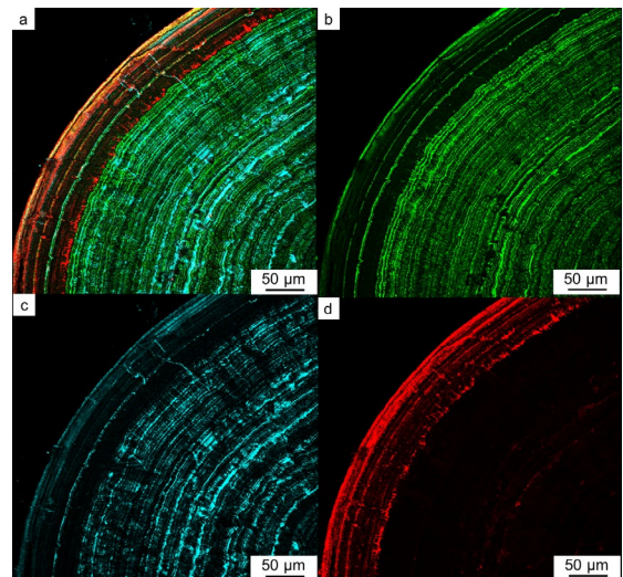
図 1 尿路結石内に分布する 3 種類のタンパク質局在の様子。(a)3 つのタンパク質の像を重ね合わせたもの。(b)オステオポンチンの分布。(c)プロトロンビンフラグメント 1 の分布。(d)カリグラニユリン A の分布。
