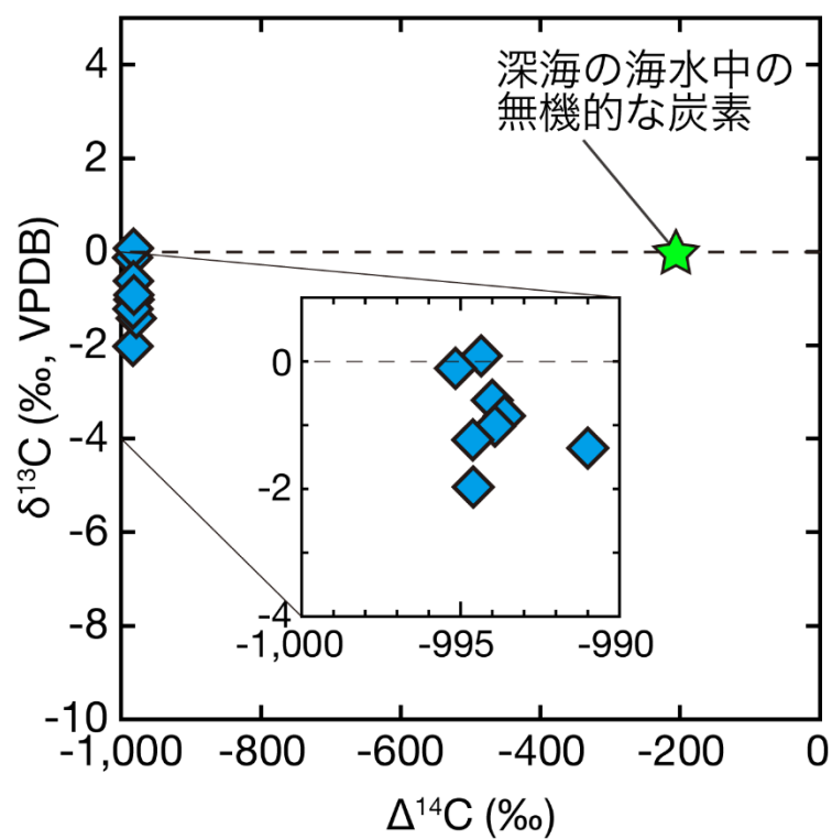
図3 炭酸塩の放射性炭素濃度 ( \Delta^{14}\text{C} ) と炭素安定同位体比 ( \delta^{13}\text{C} ) の関係を示した図。 \delta^{13}\text{C} は国際的に決められた標準試料 (VPDB) の同位体比からのずれで示される。炭酸塩に含まれる炭素は、現代の海水中に含まれる炭素とほぼ同じ \delta^{13}\text{C} 値である。一方で、現代の海水中に含まれる炭素よりも低い \Delta^{14}\text{C} 値である。
