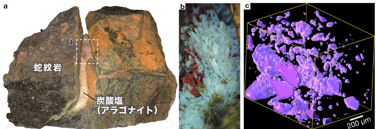
図2 (a) 炭酸塩（アラゴナイト）の産状。海亀海山の水深約 6,400m から採取した、変質したマントル岩石（蛇紋岩）の割れ目に析出している。(b) 図 2 (a) の白い点線で囲った領域の拡大図。アラゴナイトは針状の形をしている。(c) アラゴナイト脈の X 線 CT 写真。アラゴナイト脈に含まれる蛇紋岩の破片の三次元分布を示している。蛇紋岩の破片はお互いに接しておらず、流体流動と化学反応の相互作用によって炭酸塩が析出したことが明らかになった。
