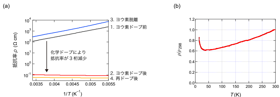
図3. 電気抵抗率の温度依存性. (a) 化学的キャリアドーピングにより金属状態になること、および、ヨウ素を脱離することで元に戻ること、さらに再度化学的ドーピングをすることで金属状態にできることが分かる. この図では横軸を温度の逆数としており、数値の小さい左端が室温（298 K）、右に行くほど低温である. (b) 金属状態は-240℃付近まで維持されている. なお、いずれの図も温度の単位としてK（ケルビン）を用いた. °Cの数値に約273を加えることでKに変換できる（例：25℃はおおよそ298 K）.
