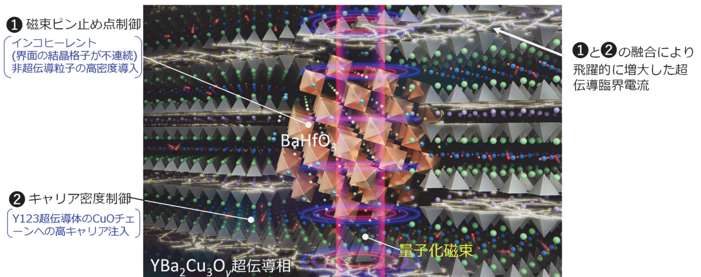
図 1 新材料設計指針により飛躍的に増大した超伝導臨界電流が YBa 2 Cu 3 O y 超伝導薄膜内を流れる様子。
