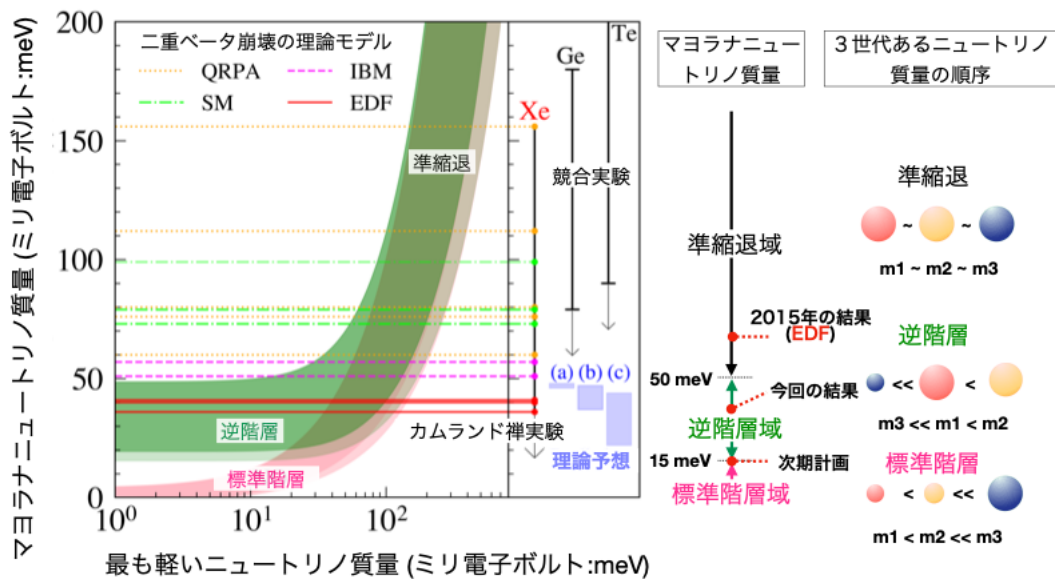
図4 今回得られたニュートリノ有効質量に対する制限
