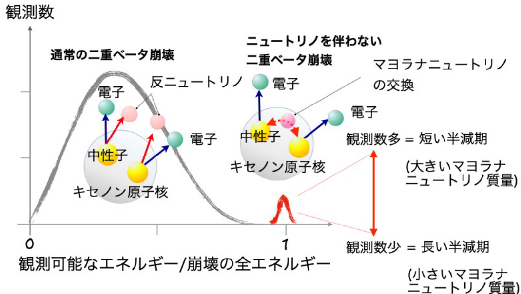
図 1 二重ベータ崩壊の説明 左側が、通常の二重ベータ崩壊で、右側がニュートリノを伴わない崩壊モードを示す。グラフの横軸は観測エネルギーを崩壊の全エネルギーで割ったもので縦軸は観測事象数。ニュートリノを伴わない崩壊モードでは、全エネルギーのところにピークが現れる(キセノン原子核の場合 2.46 MeV)。半減期が短くマヨラナニュートリノ質量が大きいと、観測数が多くなる。実験では有意な信号は確認されておらず、実験結果から半減期とマヨラナニュートリノ質量に対して制限を与えている。
