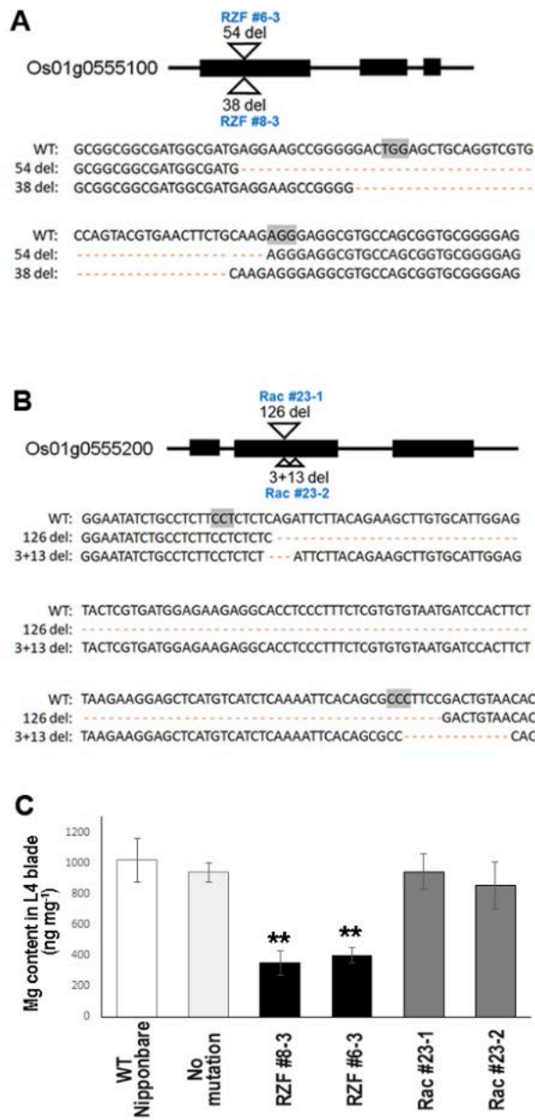
図3 2つの遺伝子 (A: Os01g0555100 (RZF)、B: Os01g0555200 (Rac)) それぞれをゲノム編集で欠損させたイネと、第四葉の葉身 (L4 blade) のマグネシウム濃度。RZFに変異を入れたイネはマグネシウム濃度が低かった。
