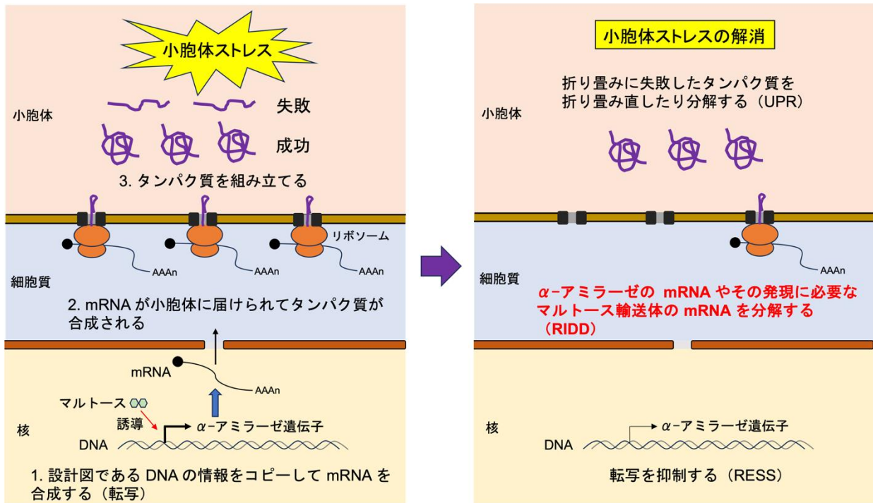
図 1 : 細菌が \alpha -アミラーゼを生産する際に起きている細胞応答機構。 \alpha -アミラーゼの生産によって誘導される小胞体ストレスの解消に RIDD が重要な役割を果たしていることが明らかとなった。
