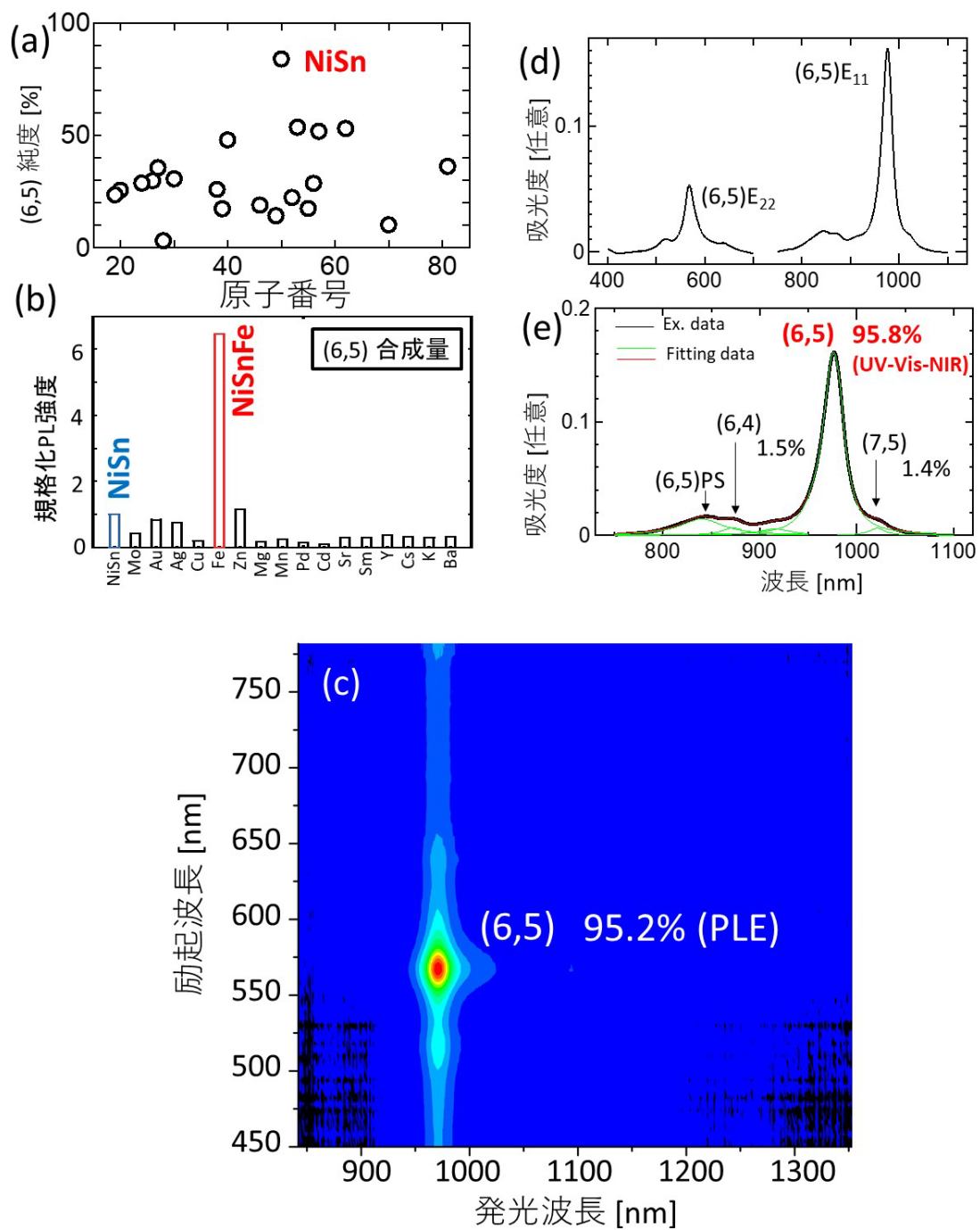
図 1 : (a)二元系触媒 (Ni+X) と(6,5)CNTs 純度の関係。二元系触媒に用いた第二因(X)の原子番号に対する(6,5)CNTs 純度のプロット図。(b)三元系触媒(NiSn+Y)と(6,5)CNTs の蛍光(PL)強度( \propto 合成量)の関係。第三因子(Y)に対する(6,5)CNTs の PL 強度依存性。(c-e) NiSnFe 三元系触媒を用いて最適合成条件で合成した CNTs の(c)蛍光-励起 (PLE) マップ、(d)紫外-可視-近赤外吸収スペクトルと(e)そのフィッティング結果。
