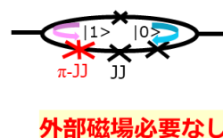
図 1 従来型と新型の超伝導磁束量子ビット回路の概念図：
