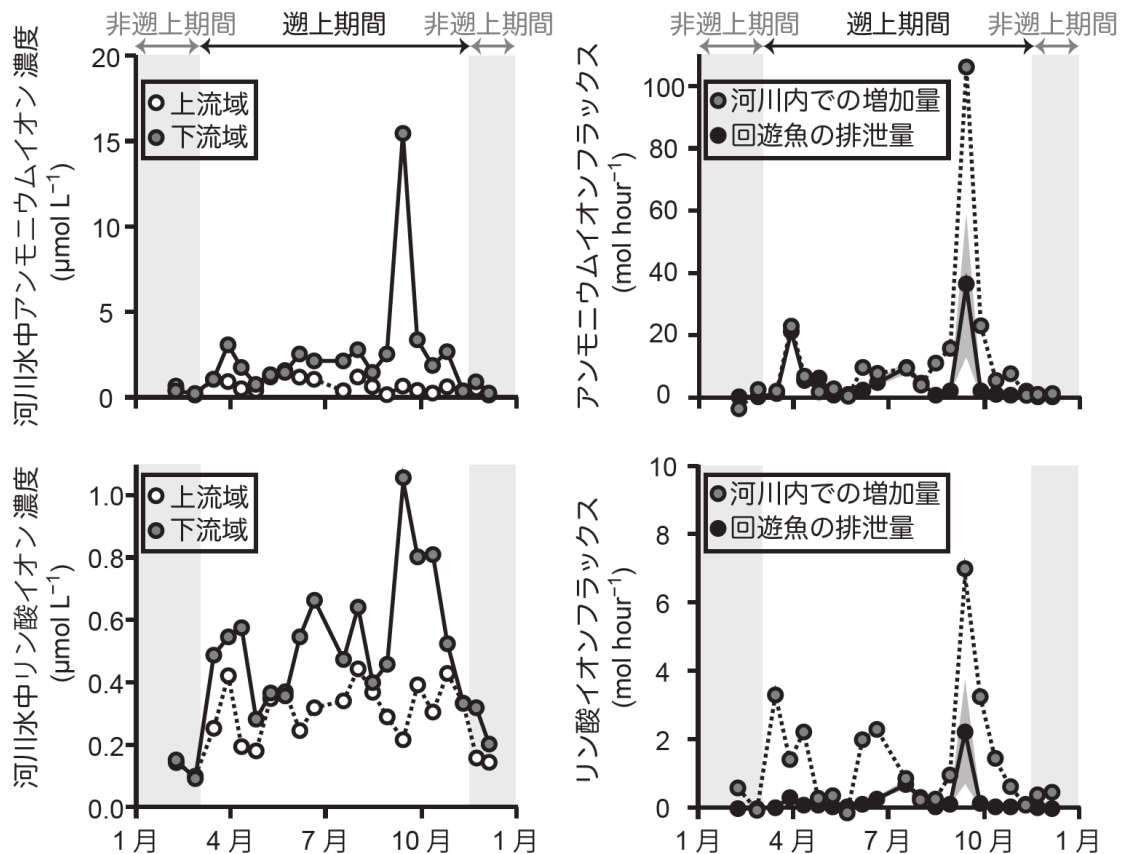
図 3. 回遊魚のいない上流域と回遊魚が多く見られた下流域の河川水で観測されたアンモニウムイオンとリン酸イオン濃度の時系列変化と河川におけるアンモニウムイオンとリン酸イオンの河川内での増加量と回遊魚による排泄投入量の時系列変化。回遊魚が見られる 8 ヶ月間の遡上期間を通して、上流域よりも下流域での濃度が高い。またアンモニウムイオンにおいては、濃度差から推定される河川での増加量は回遊魚による排泄量と良く一致している。
