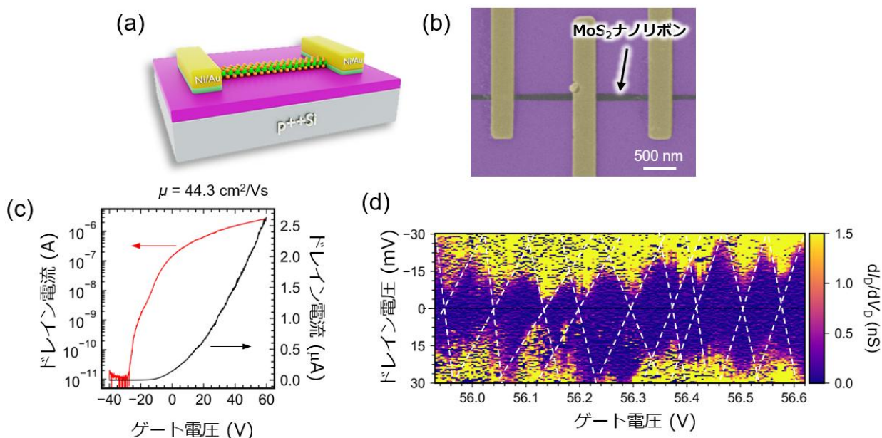
図 3 (a,b) \text{MoS}_2 ナノリボンを半導体チャネルとしたトランジスタの構造と実際の電子顕微鏡像。(c) 室温でのトランジスタ特性。(d) 極低温 (4.2 K) で得られたデバイス測定の結果。ひし形のダイヤモンドパターンが得られており、これは低次元物質特有の振る舞いとして理解される。
