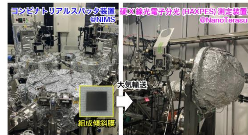
薄膜作成装置と硬X線光電子分光装置
