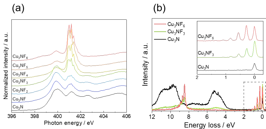
図 2 充電前後における \text{Cu}_3\text{N} 正極の N-K 吸収端での(a)X 線吸収分光測定と(b)共鳴非弾性 X 線散乱測定。(b)の挿入図は 0 eV 付近の拡大図。 \text{Cu}_3\text{N} に対して \text{F}^- を 3 mol 以上挿入した際に X 線吸収分光測定の 401 eV 付近に見られる複数のピークと共鳴非弾性 X 線散乱測定の 0 eV 付近に見られる振動ピークが分子状窒素の存在を示唆する。
