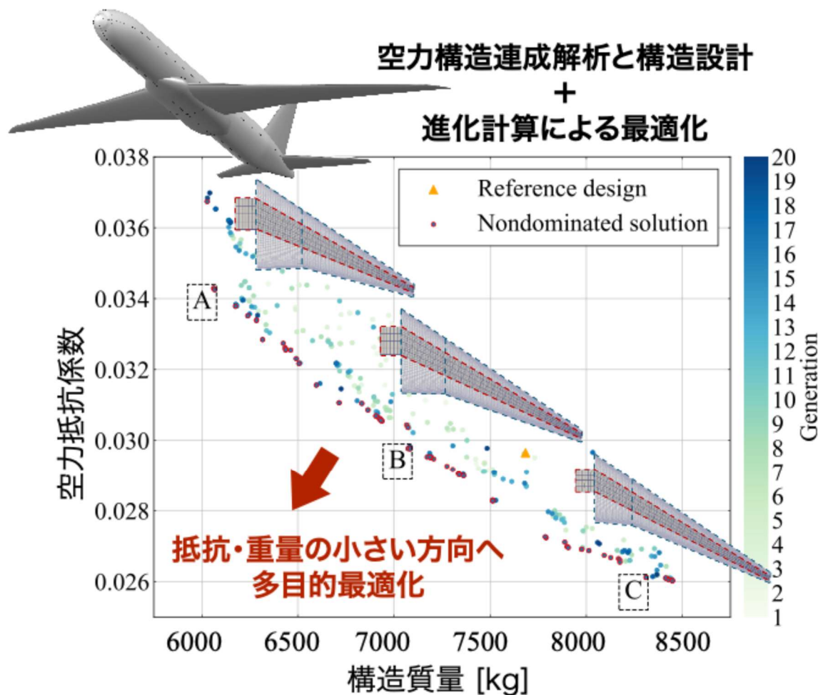
図 1. 複合材航空機主翼の空力構造最適設計（グラフの横軸は質量）
