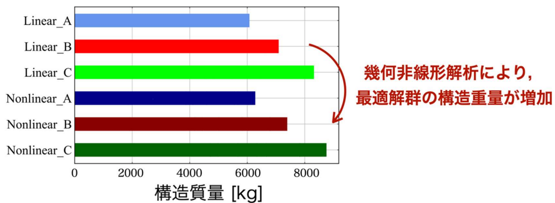
図 2. 幾何非線形解析を取り入れたことによる大変形時の構造設計重量の変化（グラフの横軸は質量）
