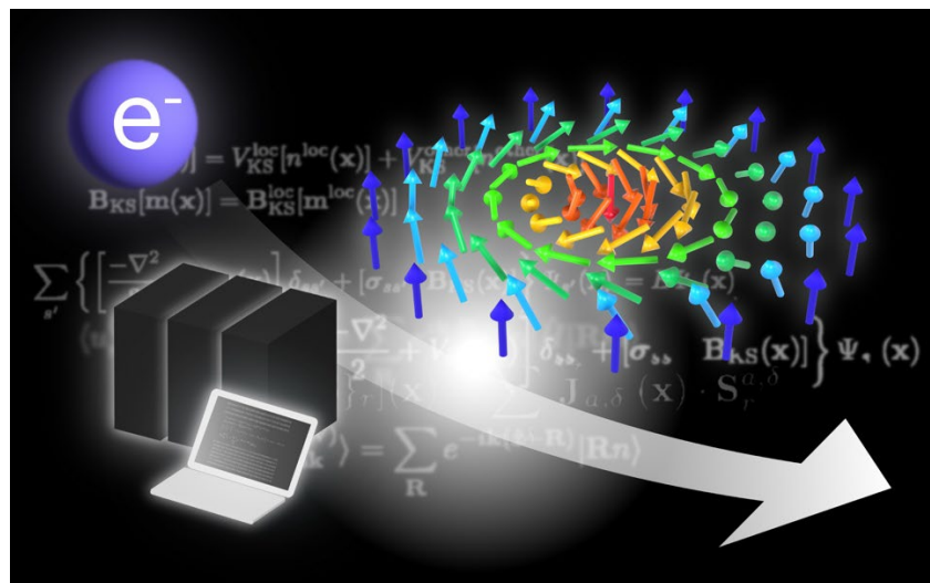
図 1. 本研究の概念図。非共面スピン構造をシミュレーションする新しい手法を開発し、通過する電子との特有な相互作用を正確に予測できるようになりました。右上の図は非共面スピン構造の一種であるスキルミオン結晶構造。
