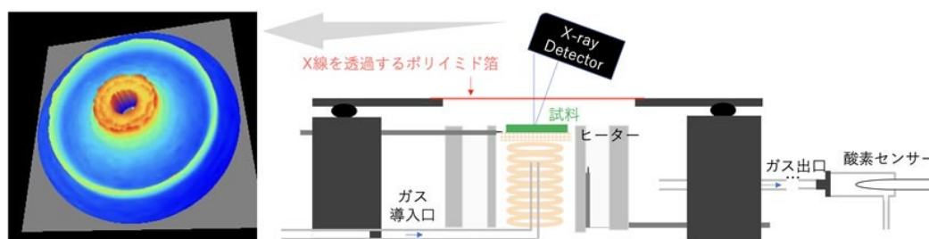
図 1. \cos \alpha 法を用いた X 線残留応力測定装置と高温測定用自作サンプルホルダの模式図。
