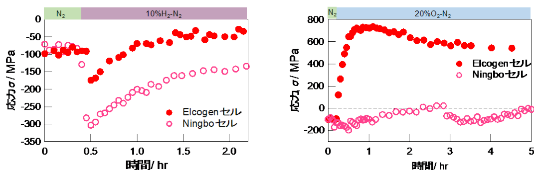
図 2. 還元（左）および酸化（右）時の YSZ 電解質応力の時間変化。負は圧縮応力、正は引張応力を示す。
