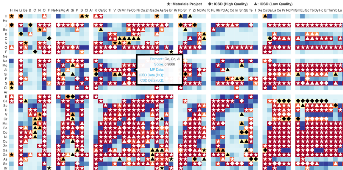
図 1 : 元素反応性マップ( https://erm.starrydata.org/ )の一部。Ge,Co,Al の 3 元系のマスにマウスを置いた状態。この例では第 1 元素をゲルマニウム (Ge) としたマップの一部を示しており、横方向が第 2 元素、縦方向が第 3 元素となっています。青色が濃い領域の一つであるコバルト (Co) とアルミニウム (Al) の組み合わせでは、データベースに登録がなかったにもかかわらず、機械学習からは高い反応性スコア 0.9866 が予測され、実験により複数の新物質の合成に成功しました。
