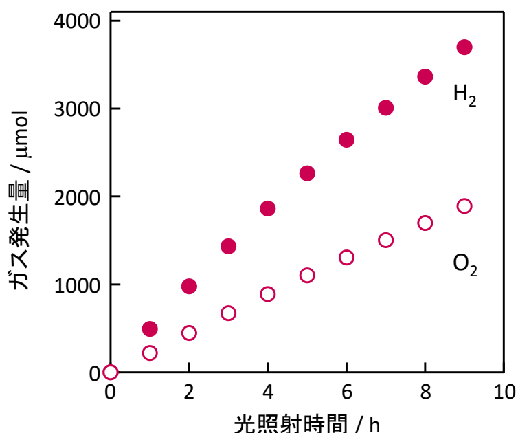
図 5. Co-HHTP を修飾した OWS 光触媒 SrTiO 3 :Al の光照射 (波長 λ > 300 nm) による H 2 および O 2 発生 の経時変化 (1 M KOH 水溶液中)。
