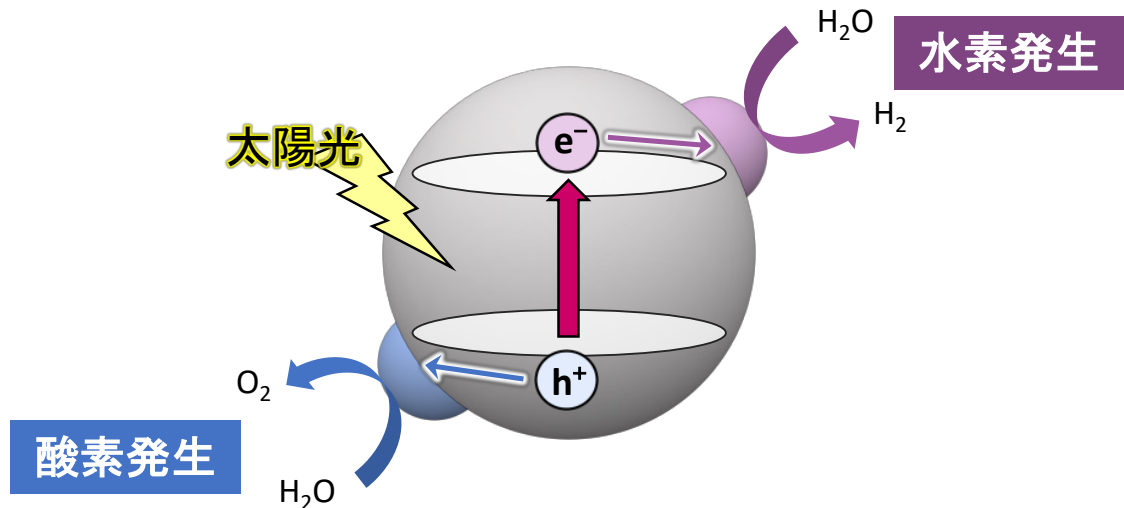
図 1. 光触媒による OWS の概念図。
