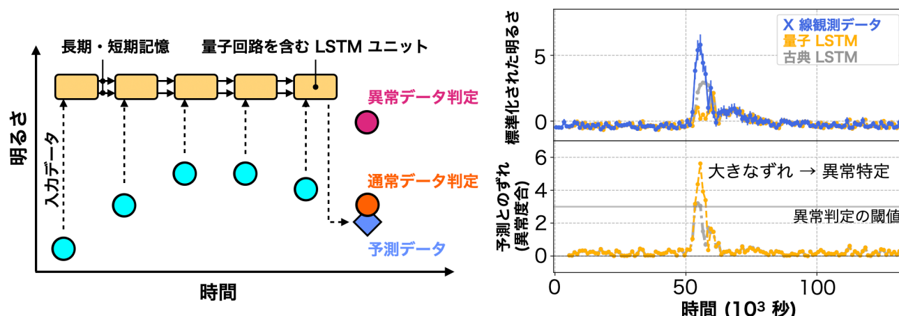
左図: 採用した量子 LSTM と異常な明るさの検知の概要。連綿と入力データを量子回路を内包した LSTM ユニットに送り、最終的に明るさを予測する(ひし形)。予測データよりも、ずれが小さい場合には通常データと判定(オレンジ丸)、ずれが大きい場合には異常現象と判定(赤紫丸)。 右図: 実際の X 線の明るさの変化に量子また古典 LSTM を適応した結果の一例。上パネルは、実際の観測データ、量子 LSTM の予測、そして古典 LSTM の予測を示している。下パネルは、観測データと予測のずれを示している。量子の方が、ずれ、または異常のシグナルが大きい。
