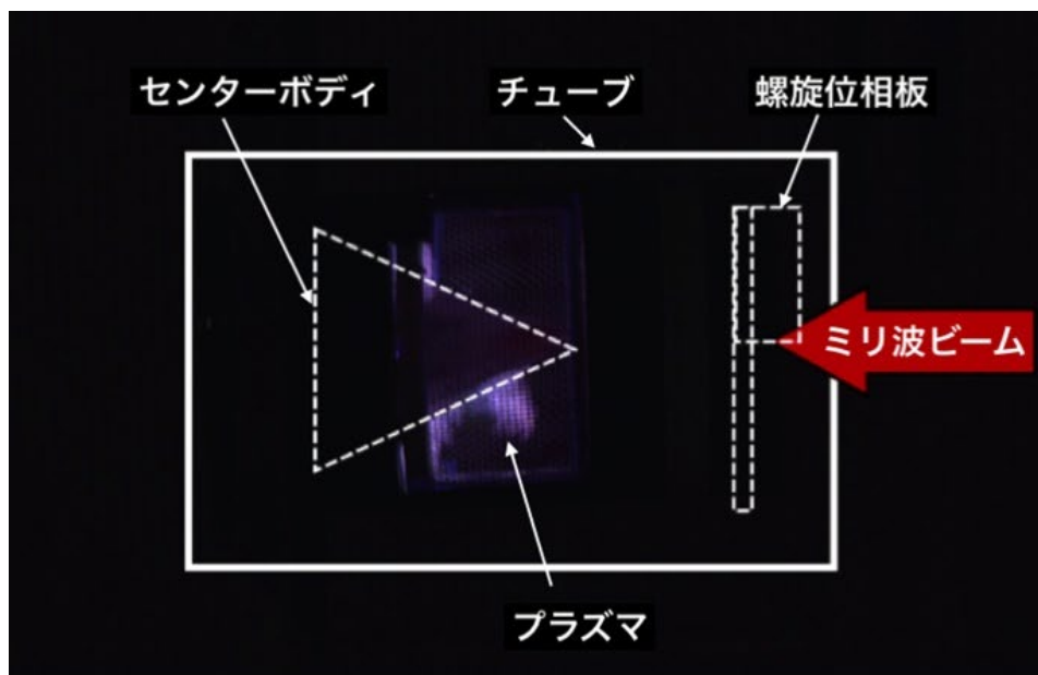
(a) 側面からの撮影写真。
