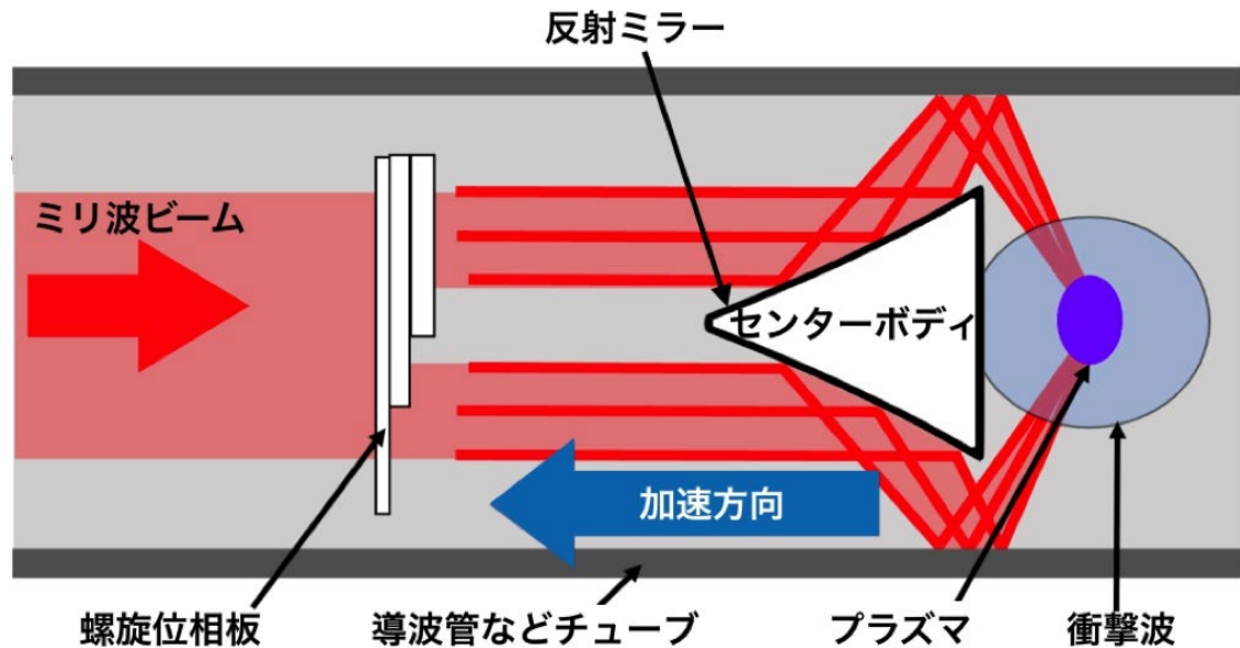
図 1. マイクロ波駆動管内加速器によるロケット打ち上げの概念図。機体前方からのミリ波ビーム照射により、チューブの中で機体を加速する。機体運動が軸方向のみに制限されるため、ビーム軸からの逸脱を避けられる。またチューブの中に気体を充填しておくことで、外気の影響を受けずに安定的に推力を生成できる。チューブはビーム伝送効率を鑑みて導波管が第一選択だが、条件によっては通常の金属チューブ、あるいは樹脂や複合材に置き換えることも考えられる。
