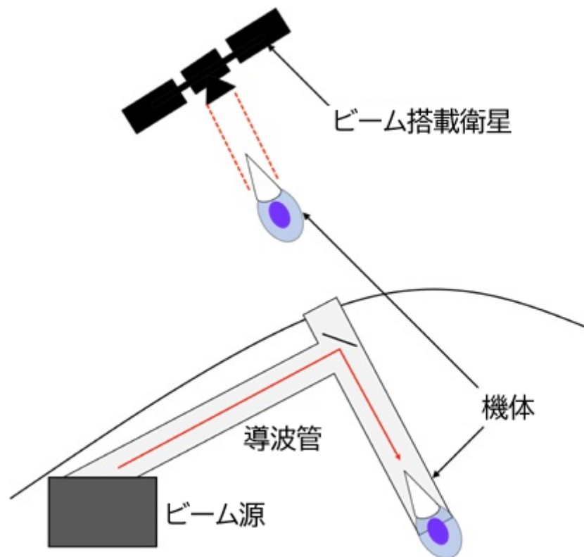
図 5. マイクロ波駆動管内加速器（MITA）の全体構想。初期加速を MITA によって与えたあとは、ビーム推進によるフリーフライトモードに移行する。
