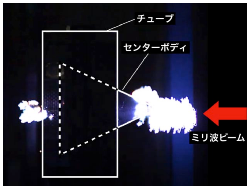
図 2. 螺旋位相板を用いない初期モデルで、原理実証に失敗した。コーン型のセンターボディ（機体）後方だけでなく、機体先端からもプラズマが生じている。機体先端で比較的強い衝撃波が駆動され、想定した推進方向とは逆向きの力が生成された。（視認性向上のため、チューブ、センターボディの輪郭を白線で補足）
