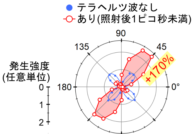
図 2. 入射光の偏光角 ( 0^\circ が分極方位) に対する、SHG 発生強度の変化。グラフの形状は結晶の対称性を反映する。テラヘルツ波を照射していないときは（青丸）四つ葉型だが、テラヘルツ波照射後（赤丸）瞬時に全く異なる形状となり、分極が傾いたことを示している。 45^\circ で観測される発生強度の増加率は 170%（元の強度の 270%）にも及び、バルク強誘電体として最大である。
