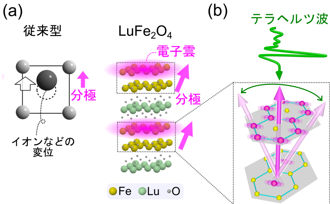
図 1. 結晶構造と本研究の実験の模式図。(a)従来型の強誘電体では重いイオンなどの変位によって分極が生じる。一方、電子強誘電体 LuFe 2 O 4 では軽い電子雲の変形によって分極が生じる。結晶構造は、鉄(Fe)原子からなる層と、Lu からなる希土類層が交互に積層している。(b)Fe 層で生じる強誘電分極と、テラヘルツ波（図中の緑矢印）による分極駆動。分極は電子（図中の紫球）のチームプレーによって生じているため刺激に敏感で、高速に制御できる。
