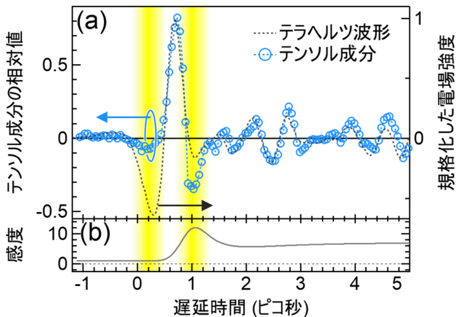
図 3. (a) テラヘルツ波形（黒点線）と、テラヘルツ波により生じた非線形光学テンソル成分 ( d_{22}^*/d_{26} ) の時間変化（青丸）。グラフ上で 0.2 ピコ秒付近では、テラヘルツ波の振幅と比べテンソル成分変化は小さい（感度が悪い）が、1 ピコ秒付近ではテンソル成分変化が大きい（感度が良い）。(b) 感度（振幅に対するテンソル成分の大きさ）の時間変化。僅か 1 ピコ秒未満で感度は約 1 桁増大する。
