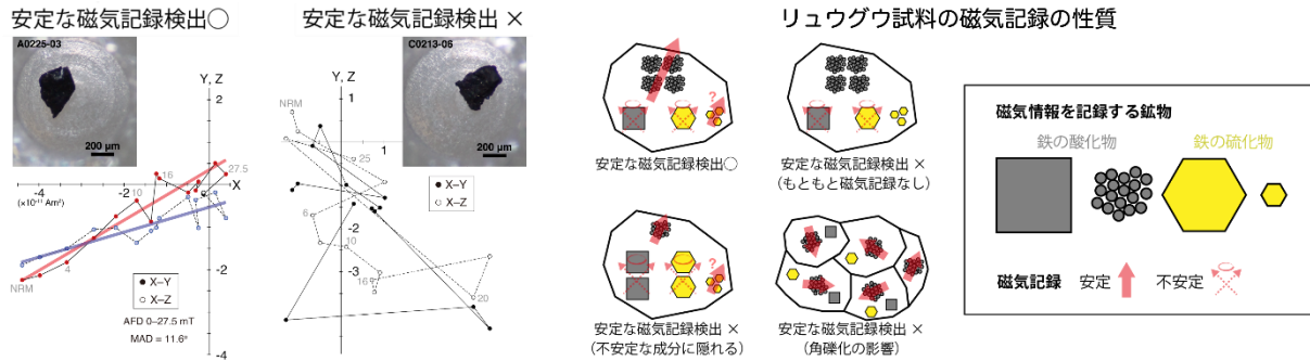
図 リュウグウ試料の磁気記録データ（左）と磁気記録の性質（右）
