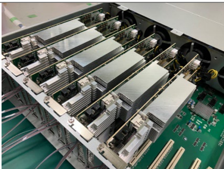
FPGA データ処理基板を収めた計算機
