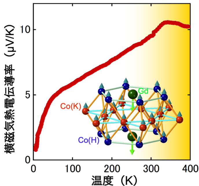
図 2： \text{GdCo}_5 における横磁気熱電伝導率の測定結果。室温(300 K)近傍において世界最大の横磁気熱電伝導率を示す。挿入図は \text{GdCo}_5 の結晶構造。ハニカム格子(H)、カゴメ格子(K)上のコバルト原子の波動関数の干渉効果により遍歴フラットバンドが生じる。
