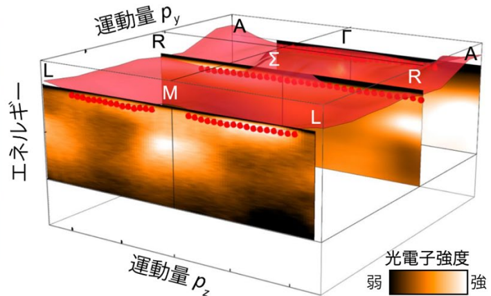
図1 (左) 積層ハニカム-カゴメ格子に配置された Co 原子による波動関数の干渉効果の模式図。 (右) 遍歴フラットバンドの角度分解光電子分光 (ARPES) による観測結果と理論計算。赤色の面が理論計算による遍歴フラットバンド、赤丸とカラーマップが ARPES により得られた遍歴フラットバンドを表す。
