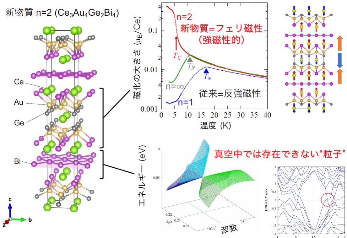
図2. 層数による磁性とトポロジカル電子状態の同時設計。今回発見した二層系物質 \text{Ce}_3\text{Au}_4\text{Ge}_2\text{Bi}_4 では、四面体層の数を増やすことで磁気秩序が反強磁性からフェリ磁性（強磁性的）へと変化するとともに、ディラック電子状態が大きく変形する。その結果、本来の相対性理論（真空中の物理）では許されない、円錐の形が限界を超えて真横に倒れ込むほど傾いた「タイプ II」という極めて異例な状態となる。
