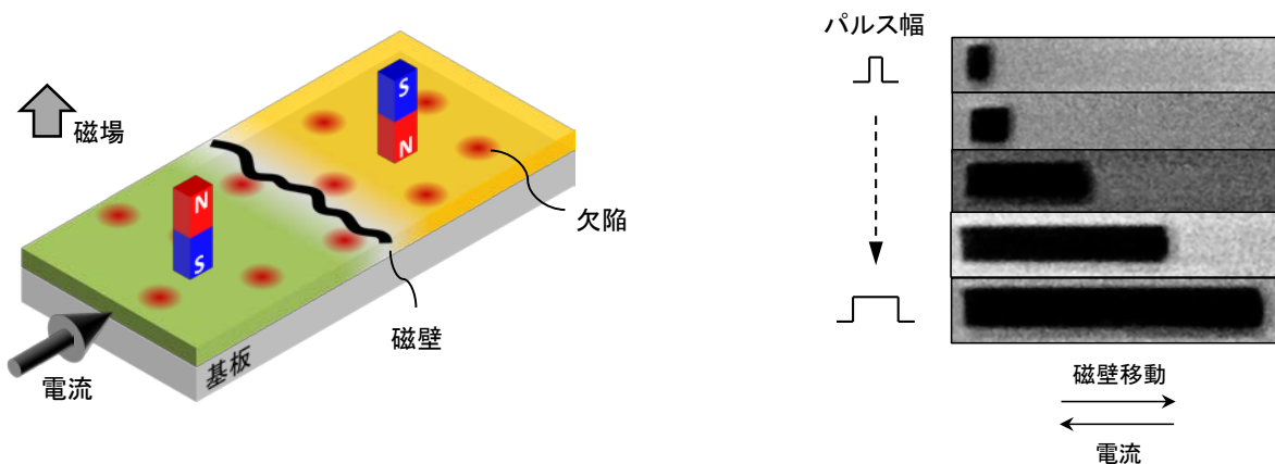
図 2：実験に用いた試料の模式図。磁化方向の異なる 2 つの磁石（磁区）の境界に形成される磁壁が試料中の欠陥に拘束されながら電流や磁場によってじわじわと一方方向に移動する（クリープ運動する）。
