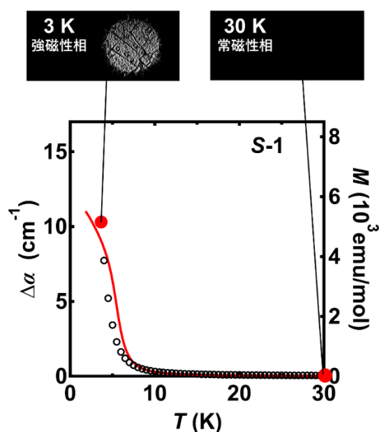
図3. 光学的電気磁気効果の観測。強磁性相(磁石になった状態)で、物質の表と裏からの透過光強度に違いが生じる。グラフ中の \Delta\alpha は光が入射する方向を変えたときの吸収係数の差、 M は試料の磁化を表している。
