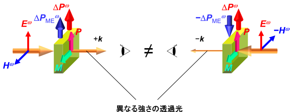
図1. 光学的電気磁気効果の概念図。電気分極( \mathbf{P} )を持つ強磁性体(極性強磁性体)では、磁性と誘電性に相関(電気磁気効果)が生じ、光(電磁波)の電場( \mathbf{E}^\omega )による電気分極( \Delta\mathbf{P}^\omega )だけでなく、磁場( \mathbf{H}^\omega )でも電気分極( \Delta\mathbf{P}_{ME}^\omega )が生じる。光が物質に入射する方向( \pm\mathbf{k} )によって、 \Delta\mathbf{P}^\omega と \Delta\mathbf{P}_{ME}^\omega の干渉の仕方が異なる為、物質を眺める方向(表裏)で明るさが異なるといった光学現象が発生する。
