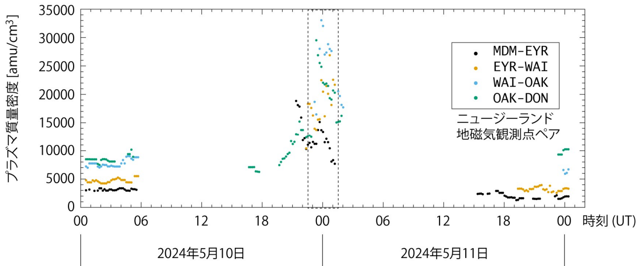
図 1 2024 年 5 月巨大磁気嵐時に観測された内部磁気圏プラズマ質量密度の増加。ニュージーランド地上磁力計ネットワークの複数観測点ペア (MDM-EYR、EYR-WAI、WAI-OAK、OAK-DON) の解析結果を示す。2024 年 5 月 10 日夜 (世界時) に、地球近傍宇宙空間においてプラズマ質量密度が急増し、特に WAI-OAK 観測点ペアでは約 35,000 amu/cm 3 に達する極端な高密度状態が観測された。破線で囲った時間帯は、「あらせ」衛星による電子密度観測と組み合わせて平均イオン質量を推定した時間帯を示す。
