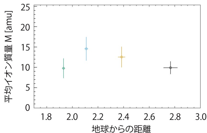
図 2 巨大磁気嵐時に推定された内部磁気圏プラズマの平均イオン質量。地上磁力計観測から推定したプラズマ質量密度と、「あらせ」衛星による電子密度観測を組み合わせることで、内部磁気圏プラズマの平均イオン質量を推定した。地球半径約 2.1-2.4 倍付近では平均イオン質量が約 15 amu に達しており、プラズマの 90%以上が酸素イオン ( O^+ ) で構成されていた可能性を示している。これは、通常の磁気嵐時に報告されている酸素イオン割合 (10-20%程度) を大きく上回る極端な状態である。
